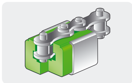
Vi har ett brett sortiment av glidskenor med integrerade bärskenor av stål, för transportör- och transmissionskedjor.
