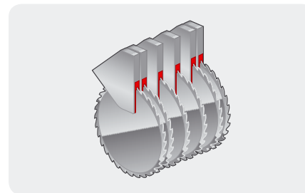
Klingstyrning av plast minskar vibrationer i sågklingan och håller den samtidigt ren.
